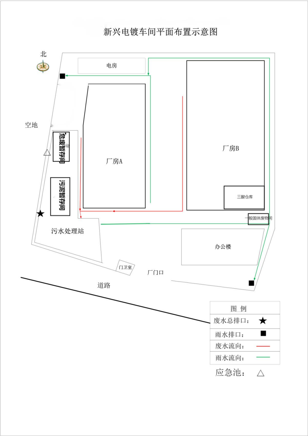
图 4.2-1 厂区平面图
