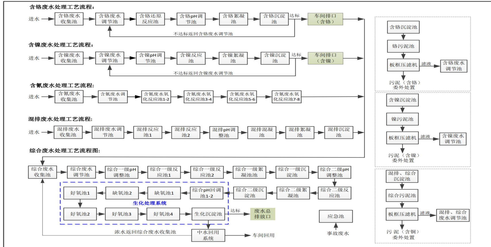
广州新兴金属有限公司电镀车间废水处理工艺流程图（2023年2月1日执行）
