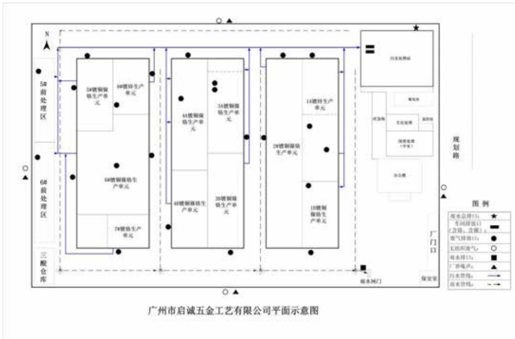
图 4.2-1 厂区平面图
