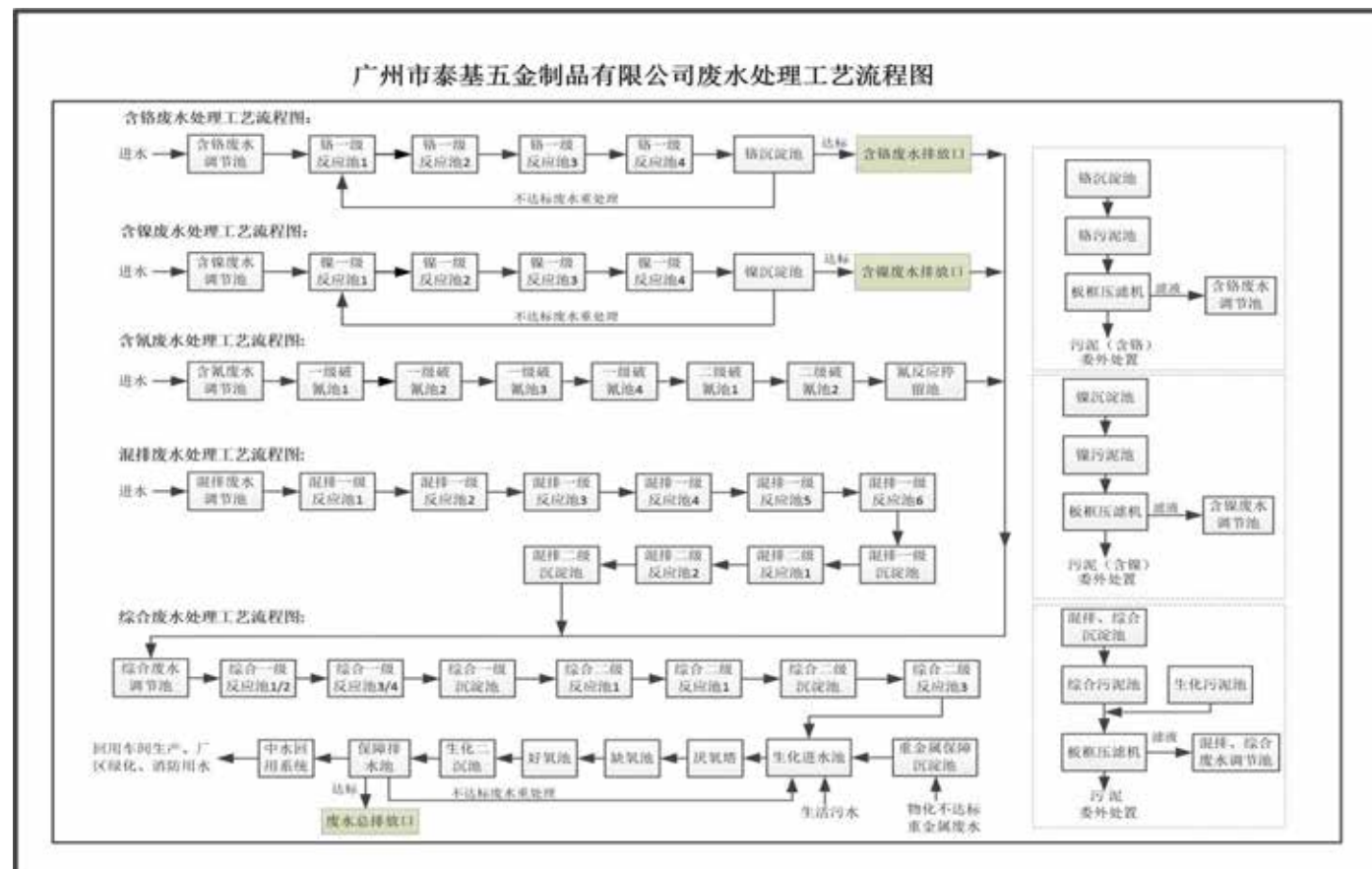
图 4.1-4 污水处理工艺流程图
