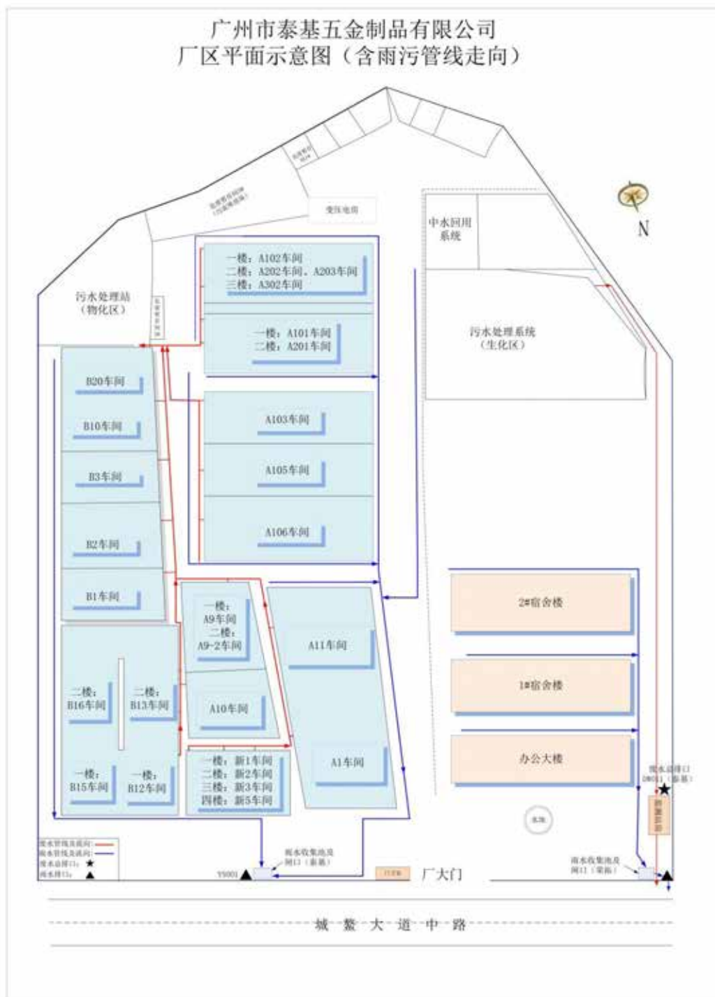
图 2.1-2 厂区平面图
