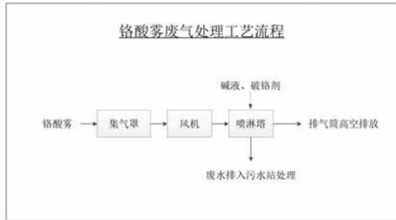
图 4.1-4 铬酸雾废气处理工艺流程图
