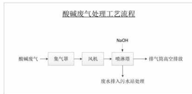
图4.1-6 酸碱废气处理工艺流程图
