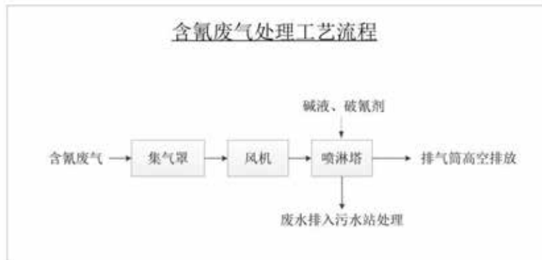
图 4.1-5 含氰废气处理工艺流程图
