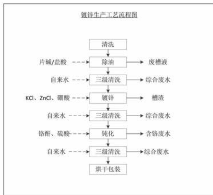
图 4.1-2 镀锌工艺流程及产污环节图
