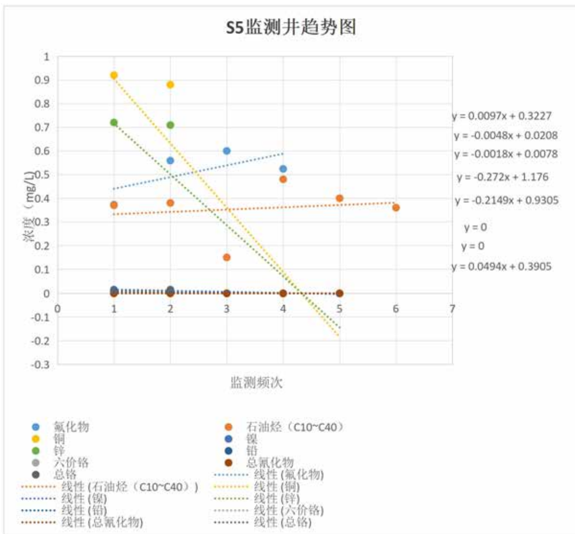
图 8.1-5 S5 监测井污染物浓度监测值变化及趋势预测
