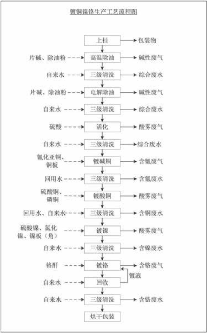
图 4.1-1 镀铜镍铬生产工艺流程及产污环节图
