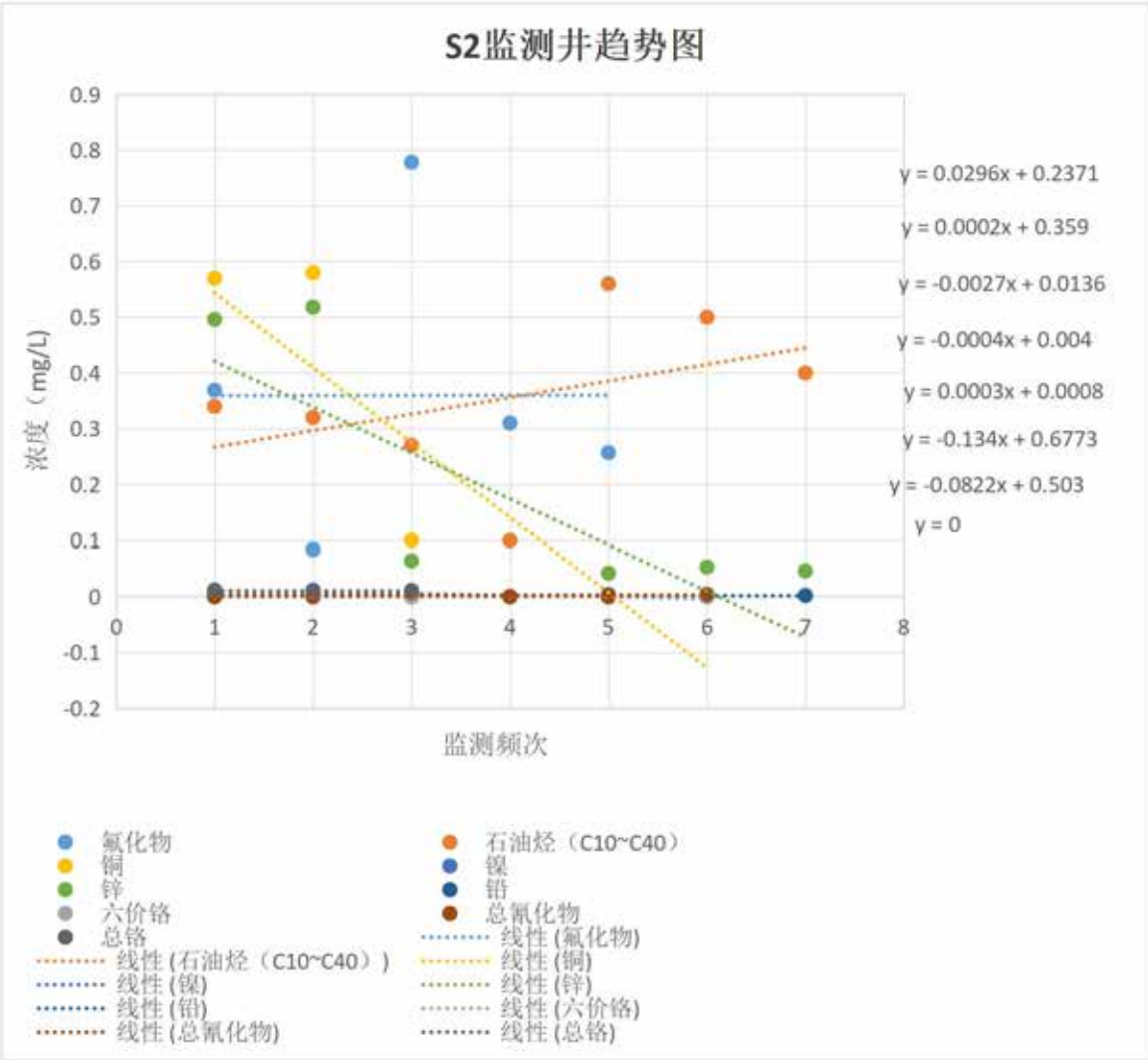
图 8.1-2 S2 监测井污染物浓度监测值变化及趋势预测
