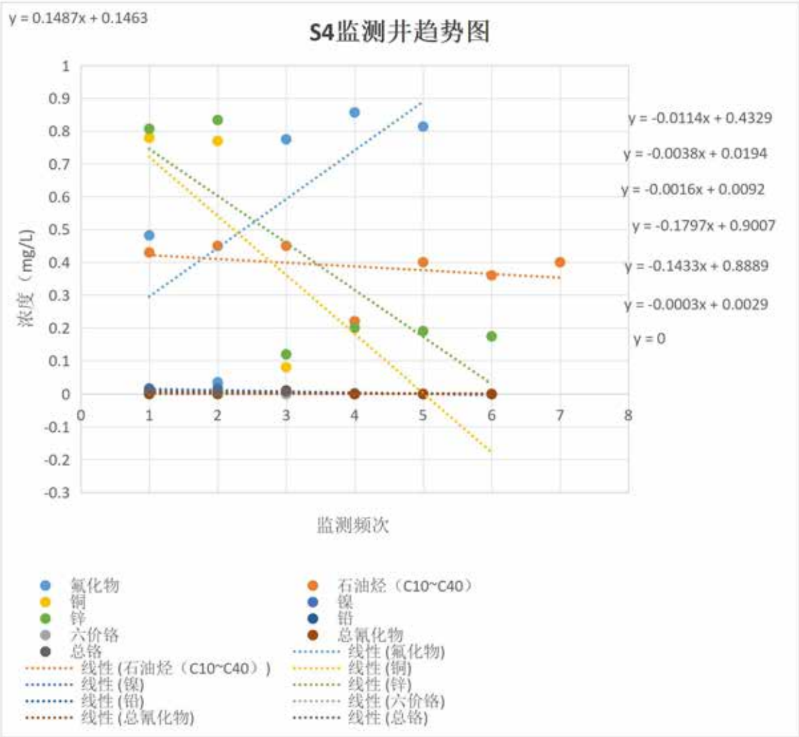
图 8.1-4 S4 监测井污染物浓度监测值变化及趋势预测
