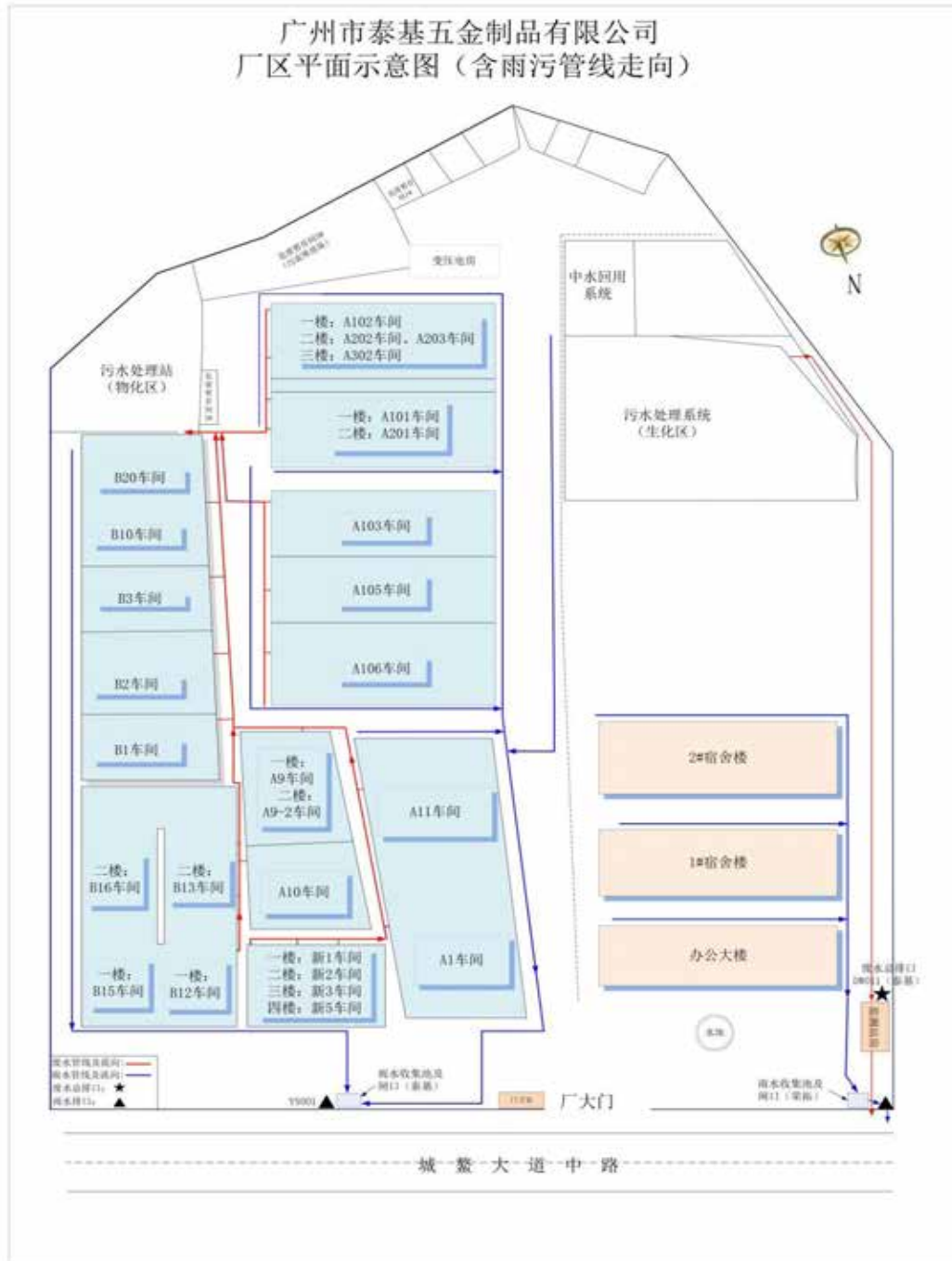
图 4.2-1 厂区平面图
