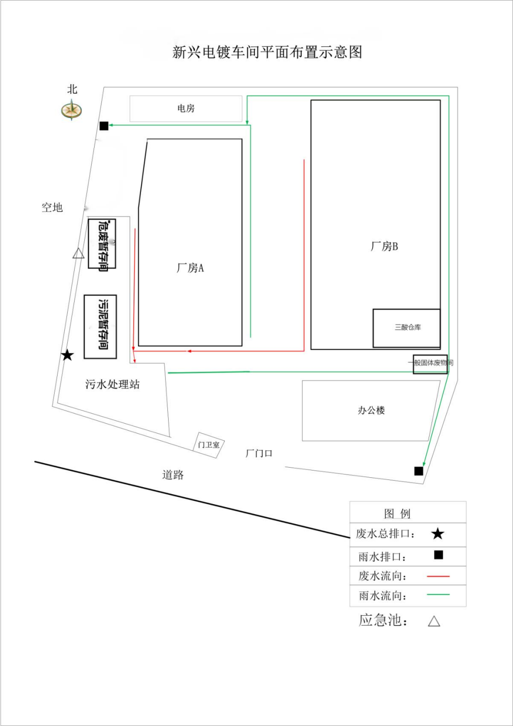
图 4.2-1 厂区平面图
