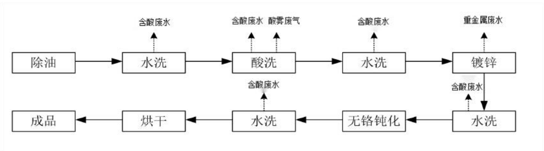
图 4.1-2 镀锌工艺流程及产污环节图
