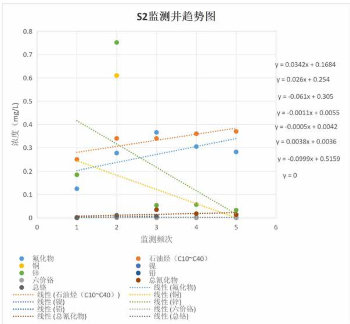
图 8.2-1 S2 监测井污染物浓度监测值变化及趋势预测
